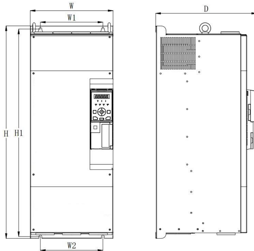
Рис. 1-4 Установочные размеры IMD183U43E ~ IMD303U43E (18.5кВт ~ 30кВт)
