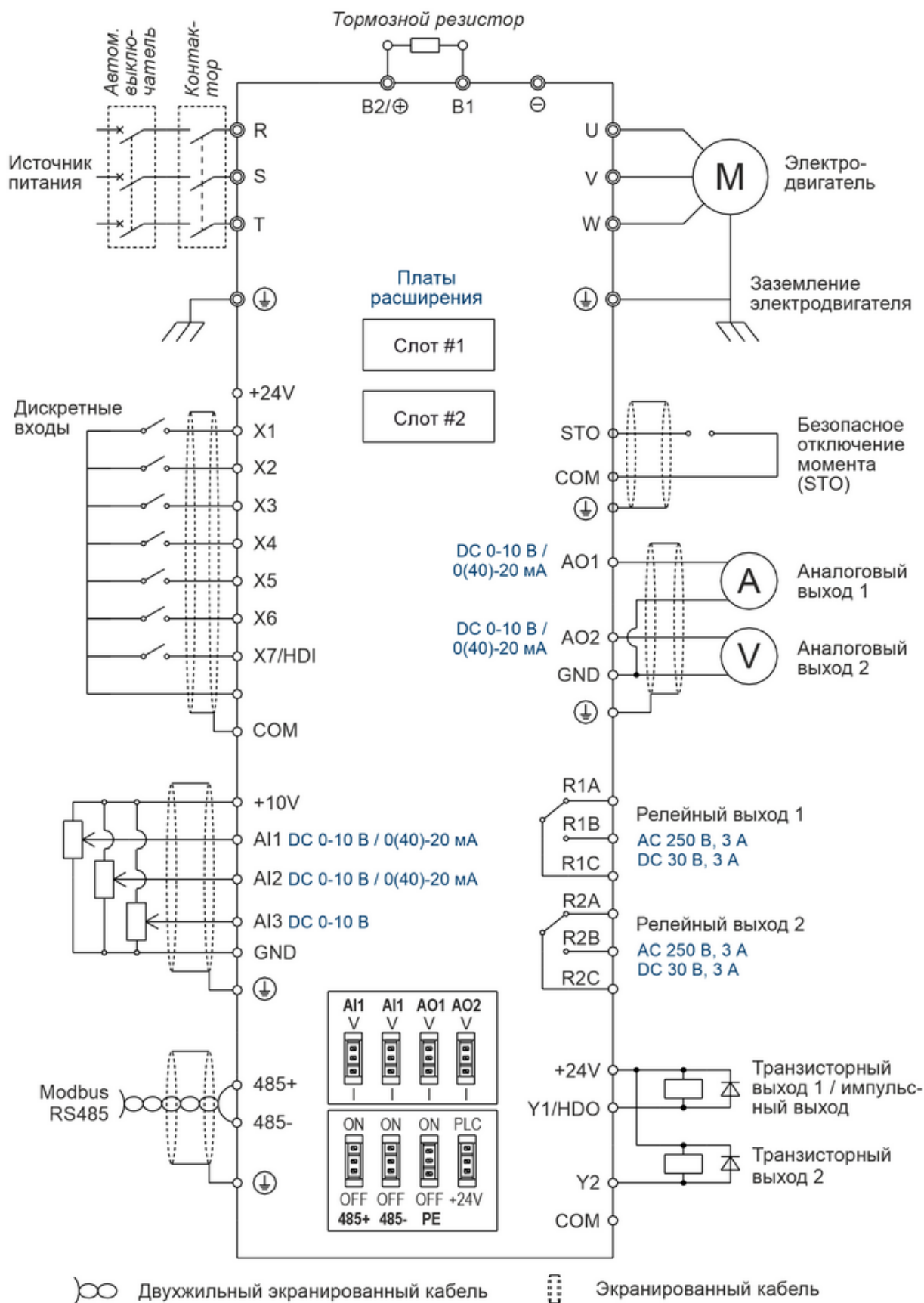
Рис. 2-4 Стандартная схема подключения
