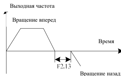
Рис. 6-6 Переключение вперед/назад
