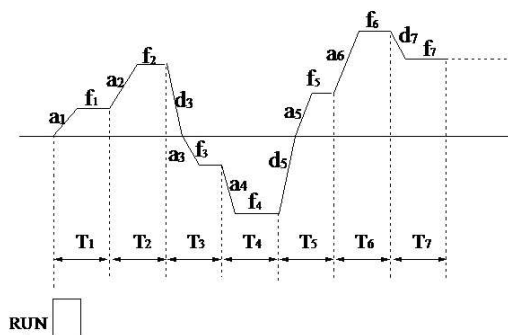
Рис. 6-25 Работа простого ПЛК
