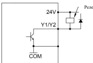
Рис. 3-12 Способ подключения внутреннего источника питания +24 В
